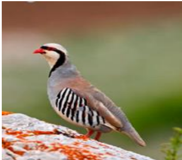
Kıvalı keklik
